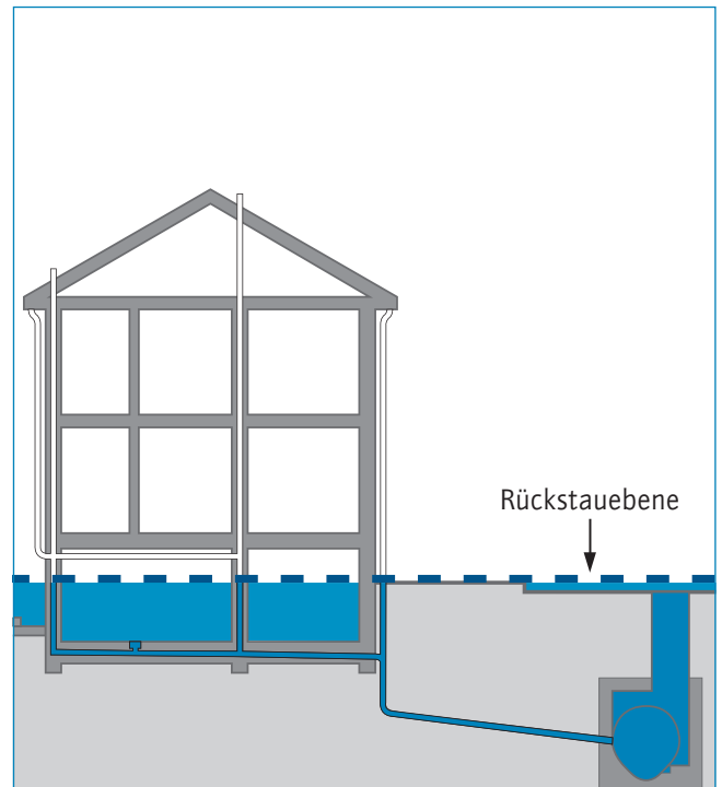
36 Rückstauenebene
