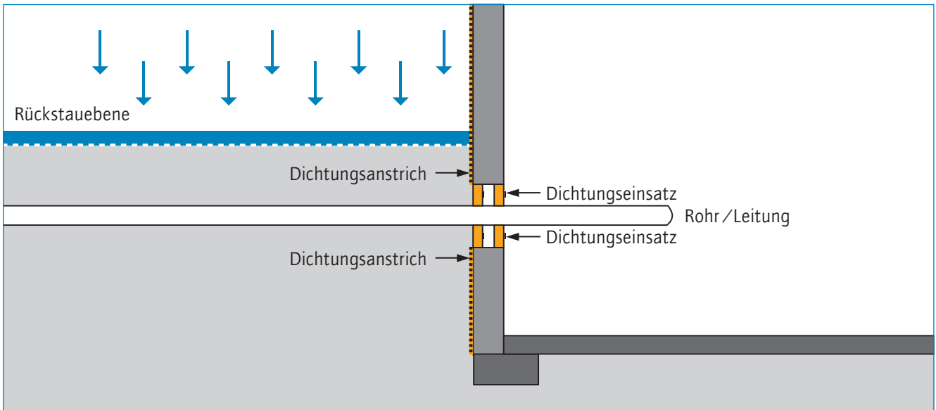
29 Abdichtung von Rohrleitungen
