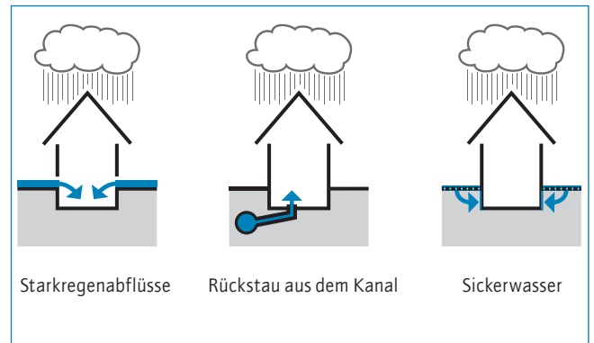
4b Überflutungsgefahren bei Starkregen
